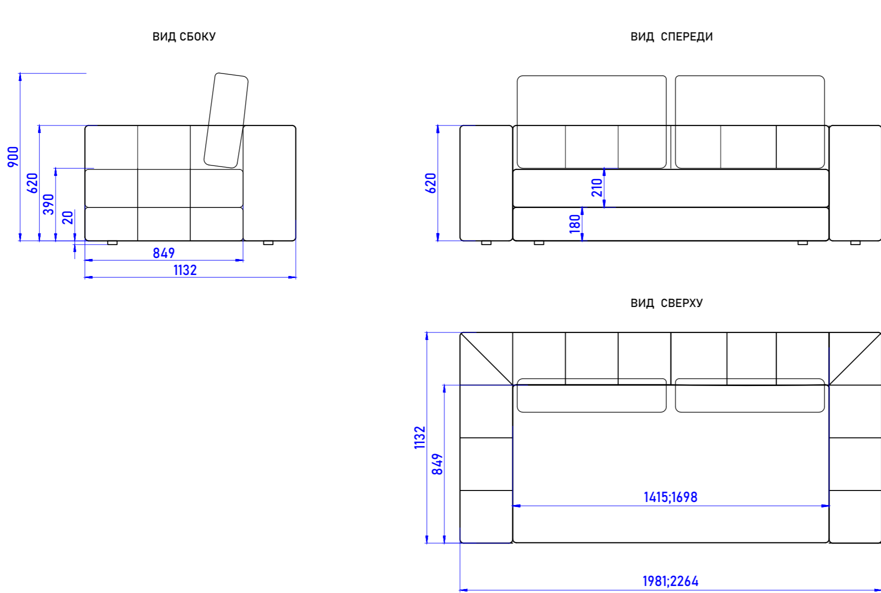
ВИД СБОКУ
