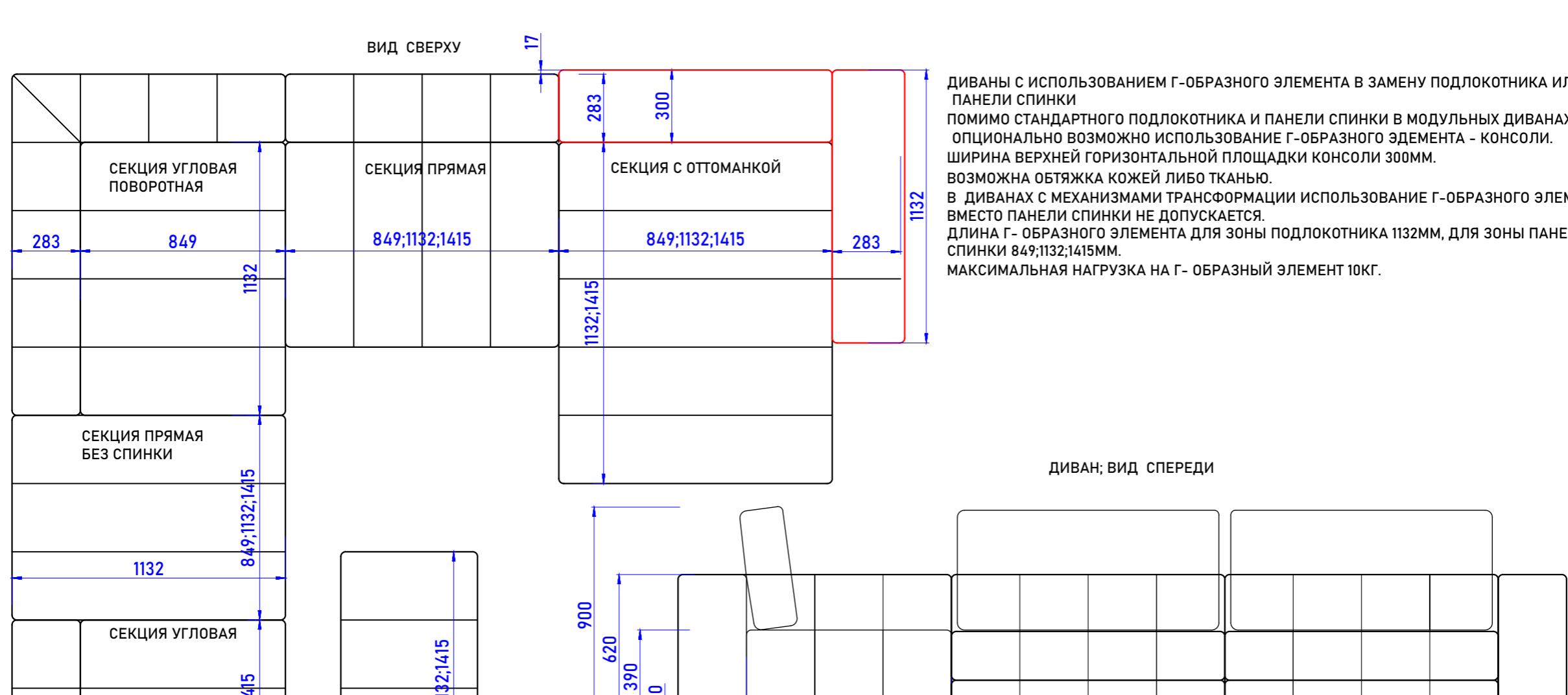
ВИД СВЕРХУ
