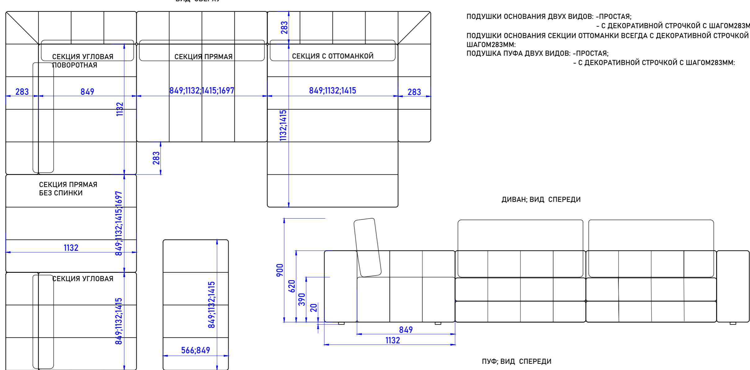
ВИД СВЕРХУ
